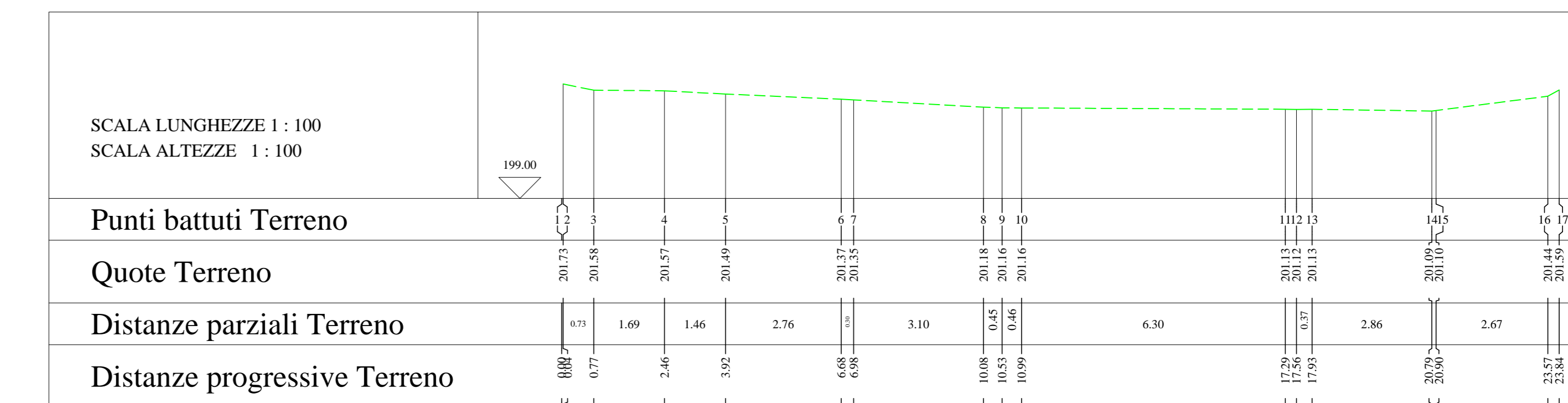
PROFILO N°4
